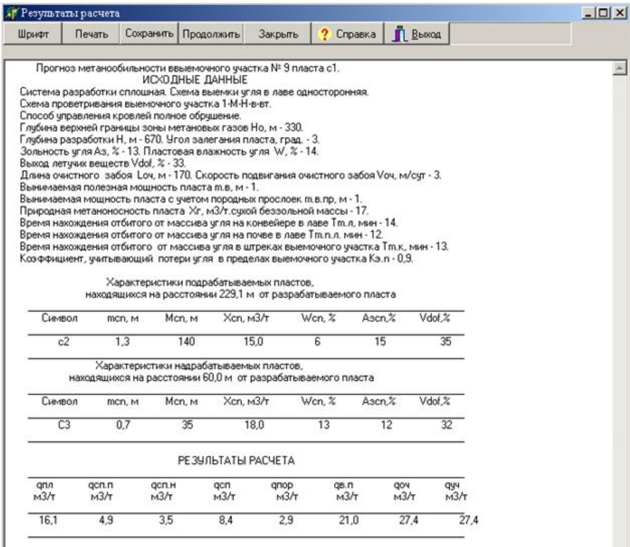
Рис. 3. Вікно результатів розрахунку
