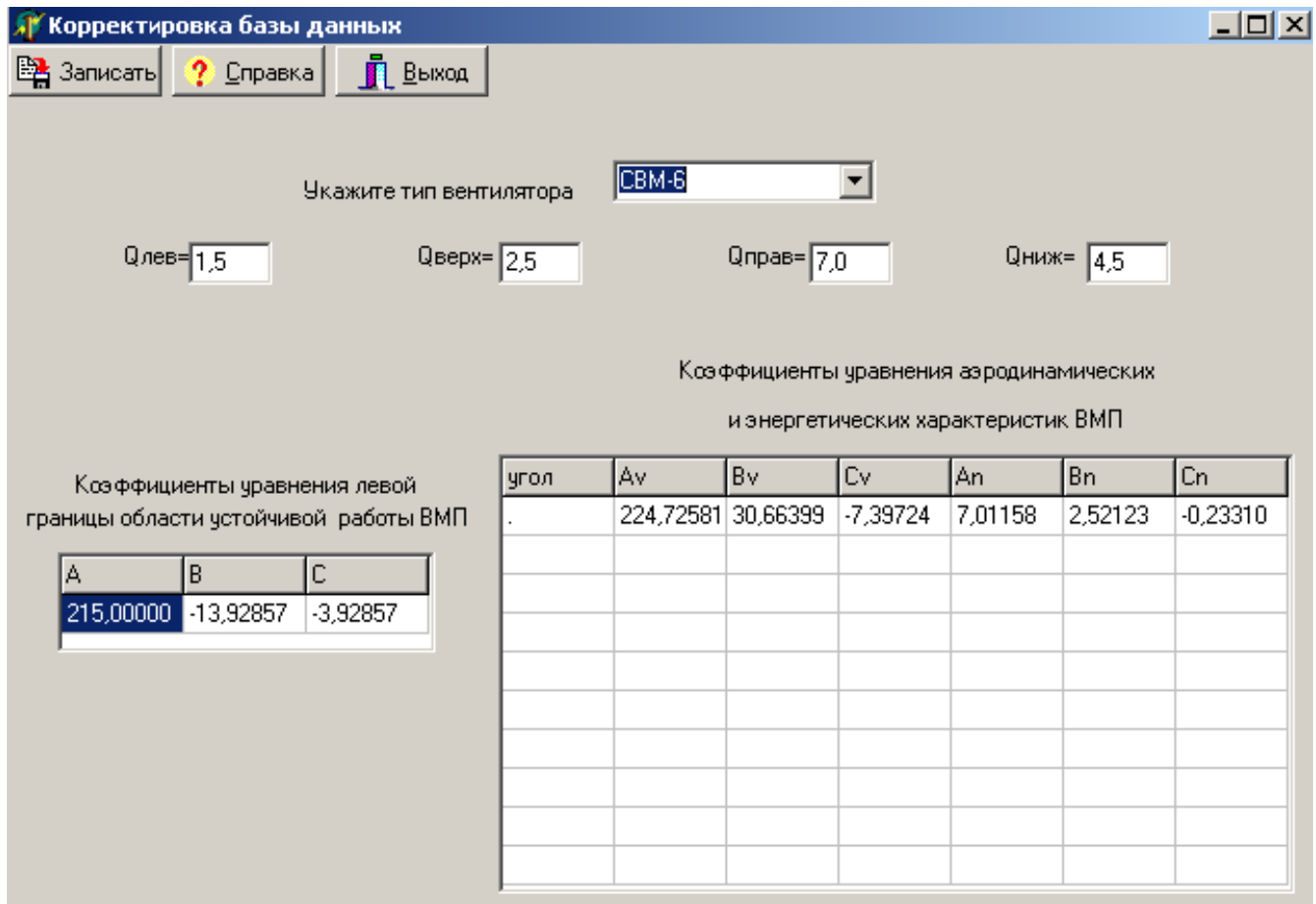
Рис. 18. Вікно коректування бази даних ВМП
